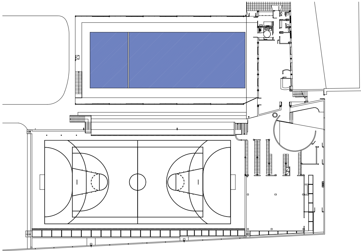
PLANTA BAJA
